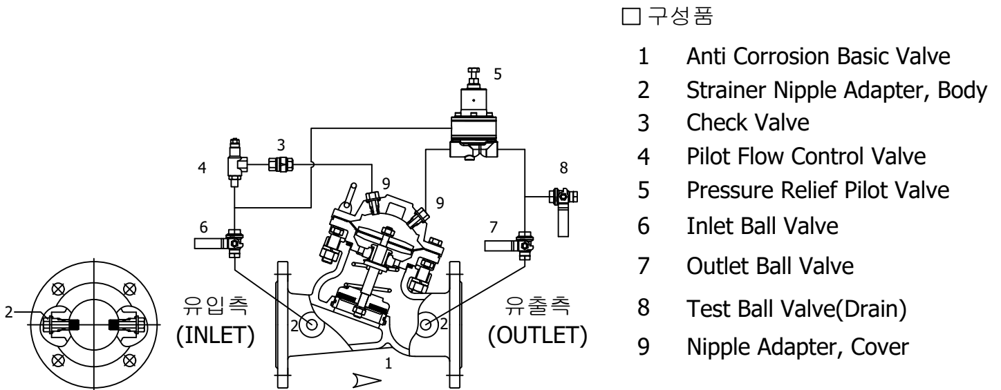
그림 3 부식방지 파일럿 식 릴리프 및 압력유지밸브(W02-010-AC)의 제어 배관도
